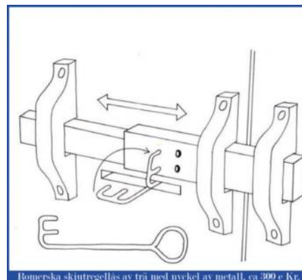
Bomerska skjutregellås av trä med nyckel av metall, ca 300 e Kr.
