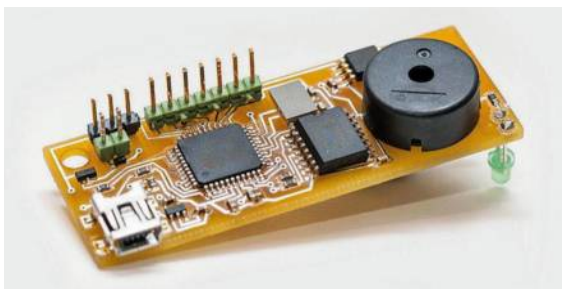
Elektronikenheten TAC.
